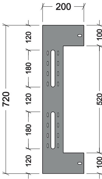
PROSPETTO LATERALE
