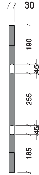
PROSPETTO POSTERIORE
