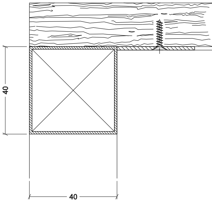
SISTEMA DI FISSAGGIO TOP TAVOLO
