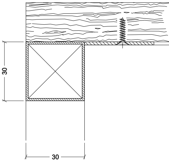
SISTEMA DI FISSAGGIO TOP TAVOLO
