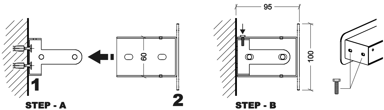
SISTEMA DI FISSAGGIO A PARETE
