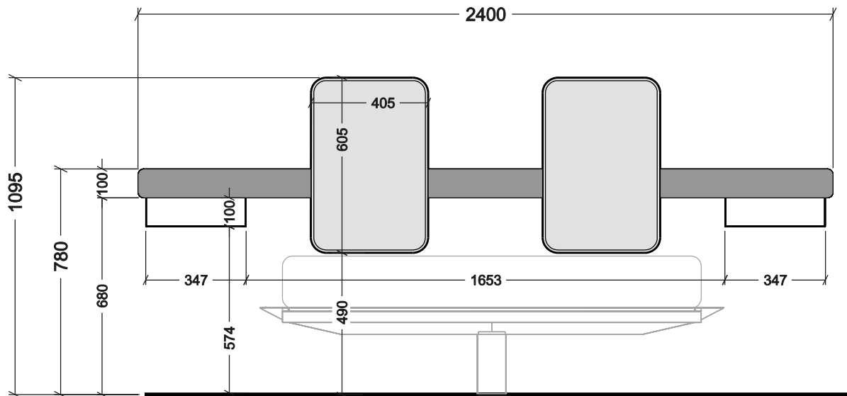
PROSPETTO FRONTALE
