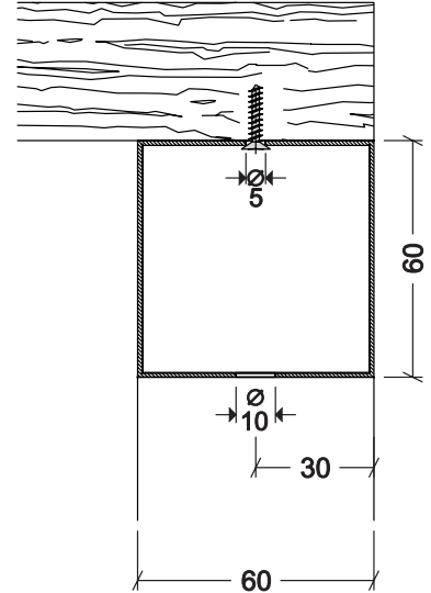
SISTEMA DI FISSAGGIO AL PIANO DELLA PENISOLA
