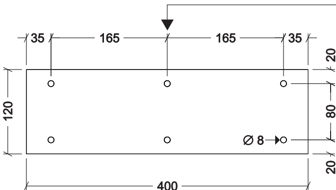
PIASTRA SPESSORE 3 mm. SALDATA FILO SUPERIORE DELLA GAMBA
