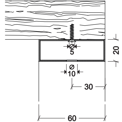
SISTEMA DI FISSAGGIO AL PIANO DELLA PENISOLA
