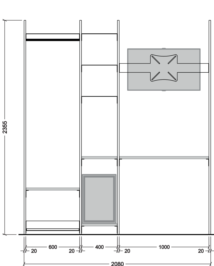
PROSPETTO FRONTALE
