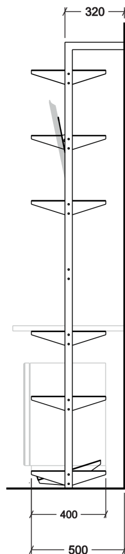
PROSPETTO LATERALE
