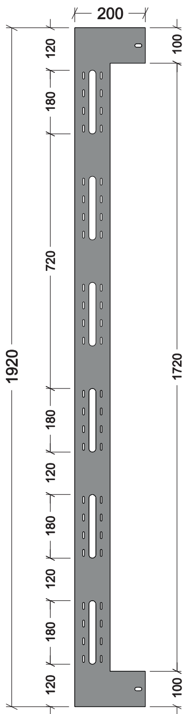
PROSPETTO LATERALE
