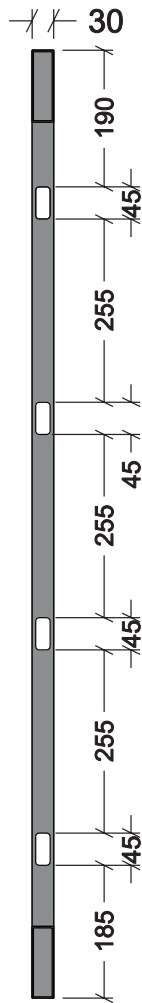
PROSPETTO POSTERIORE
