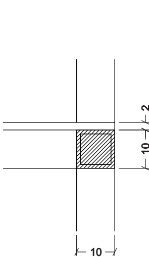
PARTICOLARE POSIZIONE RIPIANO
